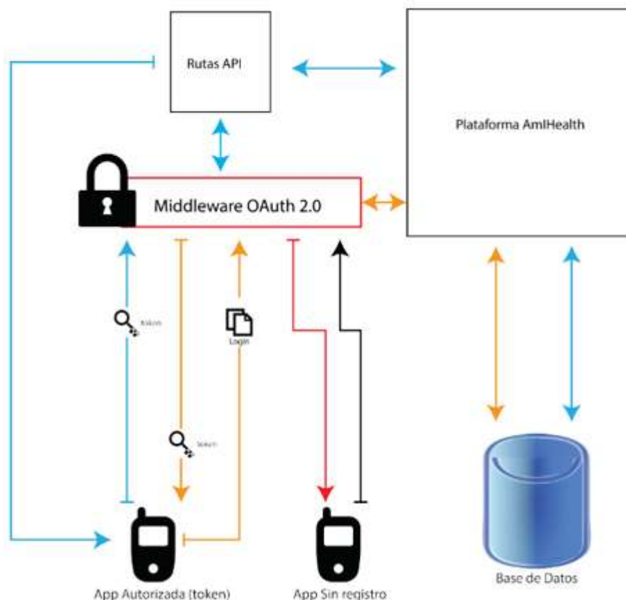
Fig. 5 - Arquitectura de servicio AmiHEALTH .
