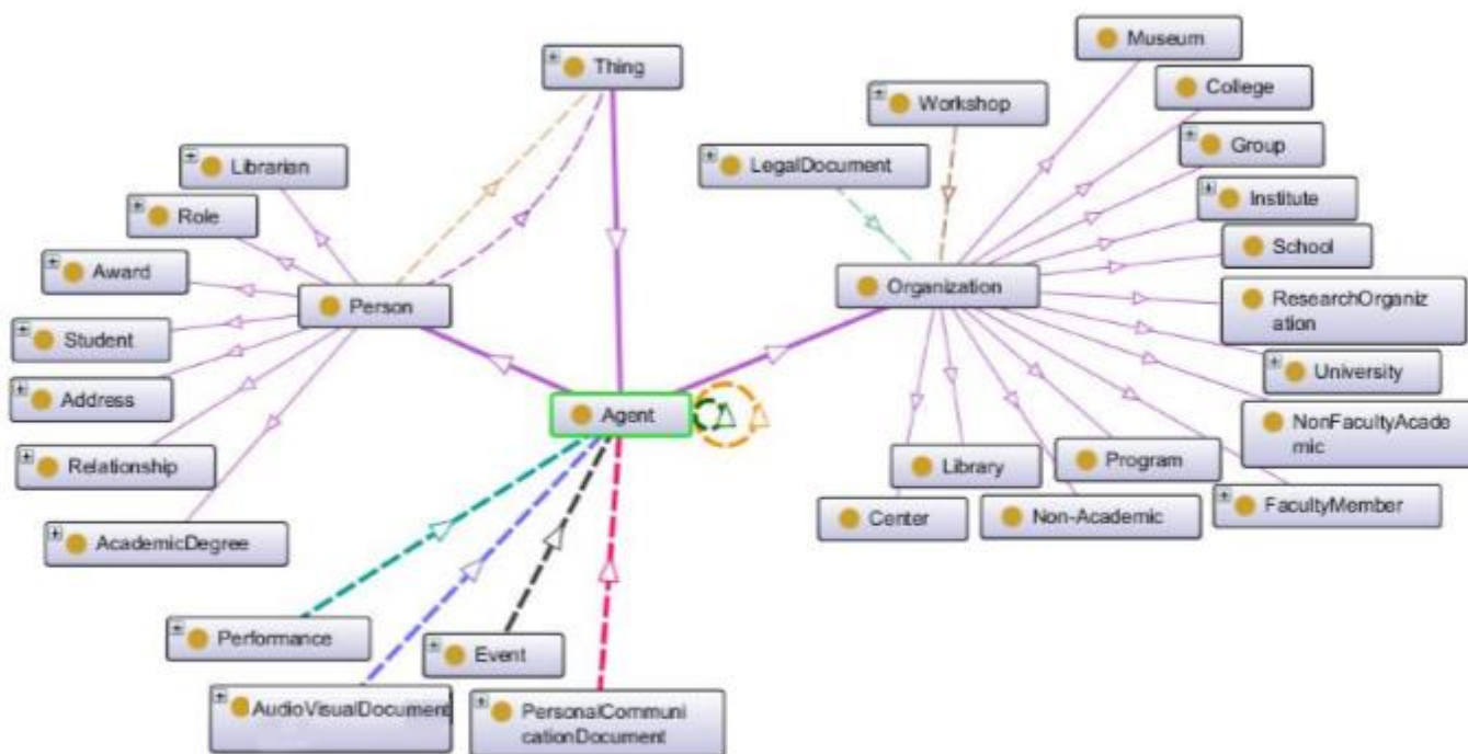
Fig. 1. UH ontology: Clase Agente y su relación con otras clases y subclases de la ontología. Visualización desde Protegé.
